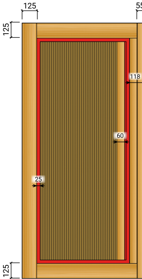
Largeurs de frise minimales, pour panneaux bruts NON raccourcis en mm
