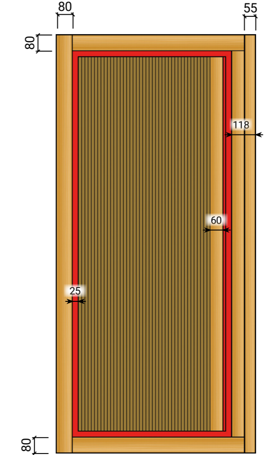
Largeurs de frise minimales, pour panneaux bruts NON raccourcis en mm
